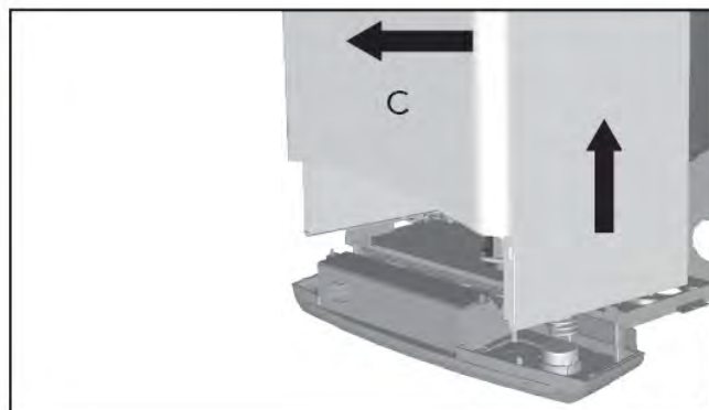
рис. 9 - Демонтаж кожуха
