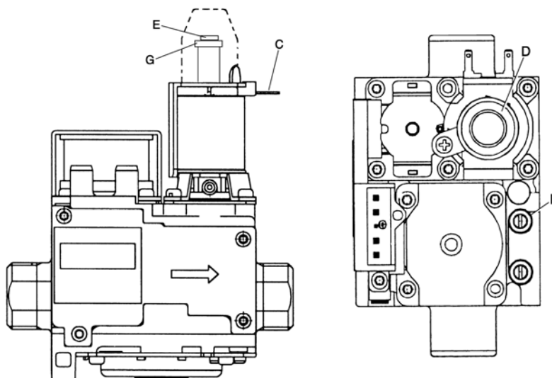
рис. 8 - Газовый клапан
