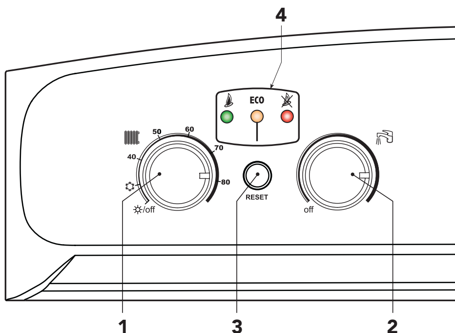
рис. 1 - Панель управления
